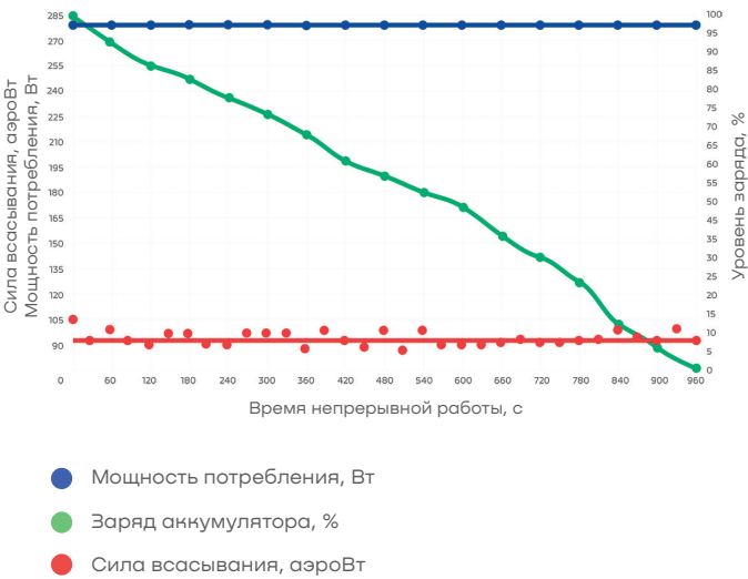
График измерения мощности в режиме Turbo+**
